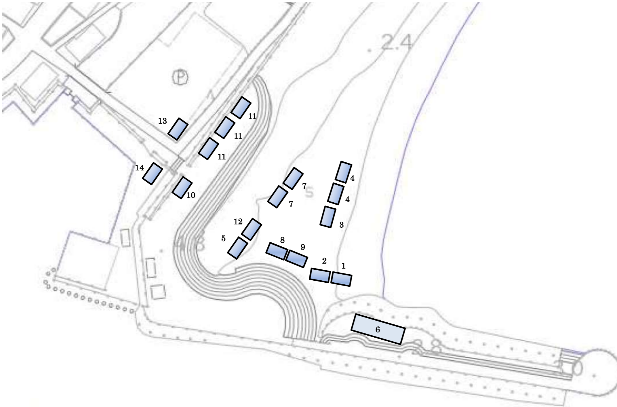
尾鷲市三木里海岸OWS会場 テント配置予定図 (1/1500) 図-1
